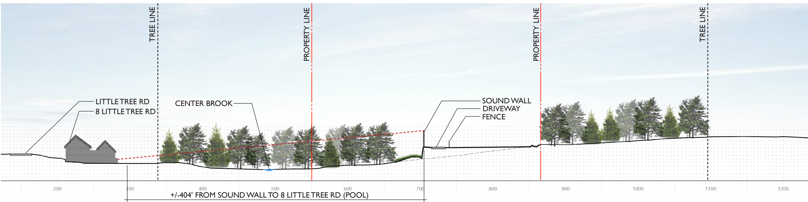
SECTION A-A
